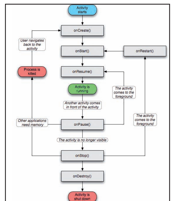
Fig. 1: State Diagramm che illustra il Life Cycle di un'activity
