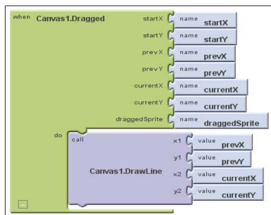
Fig. 17: La logica per tracciare una linea ad ogni movimento del dito sul componente “Canvas1”
