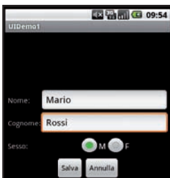
Fig. 19: Una maschera di immissione dati realizzata combinando più widget e più layout
