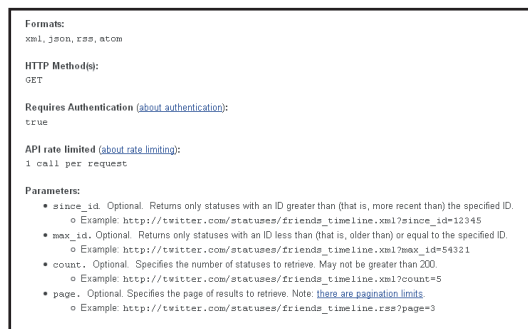
Fig. 1: Formato di una request per ottenere la friends-timeline dello user specificato nella fase di autenticazione
