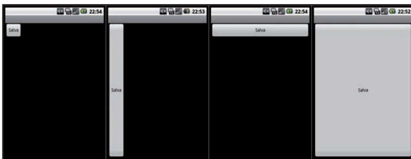
Fig. 4: Dimensionare un componente rispetto al suo contenitore. Da sinistra a destra: wrap_content su layout_width e layout_height ; wrap_content su layout_width e fill_parent su layout_height ; fill_parent su layout_width e wrap_content su layout_height ; fill_parent su layout_width e su layout_height .
